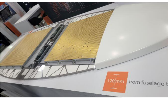
한화페이저 평판형 안테나
