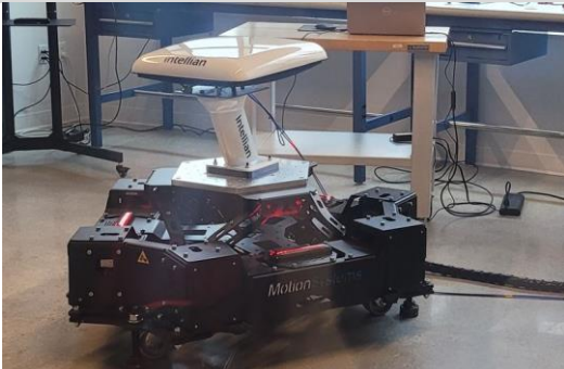
인텔리안테크 ADC센터, 평판형 안테나 진동테스트
